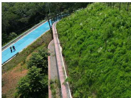
<배수로 전경>
